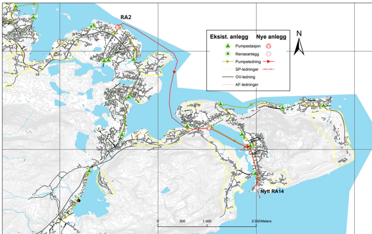
Overføring frå RA2 Fiskarstrand til nytt reinseanlegg RA14 ved Sunde
