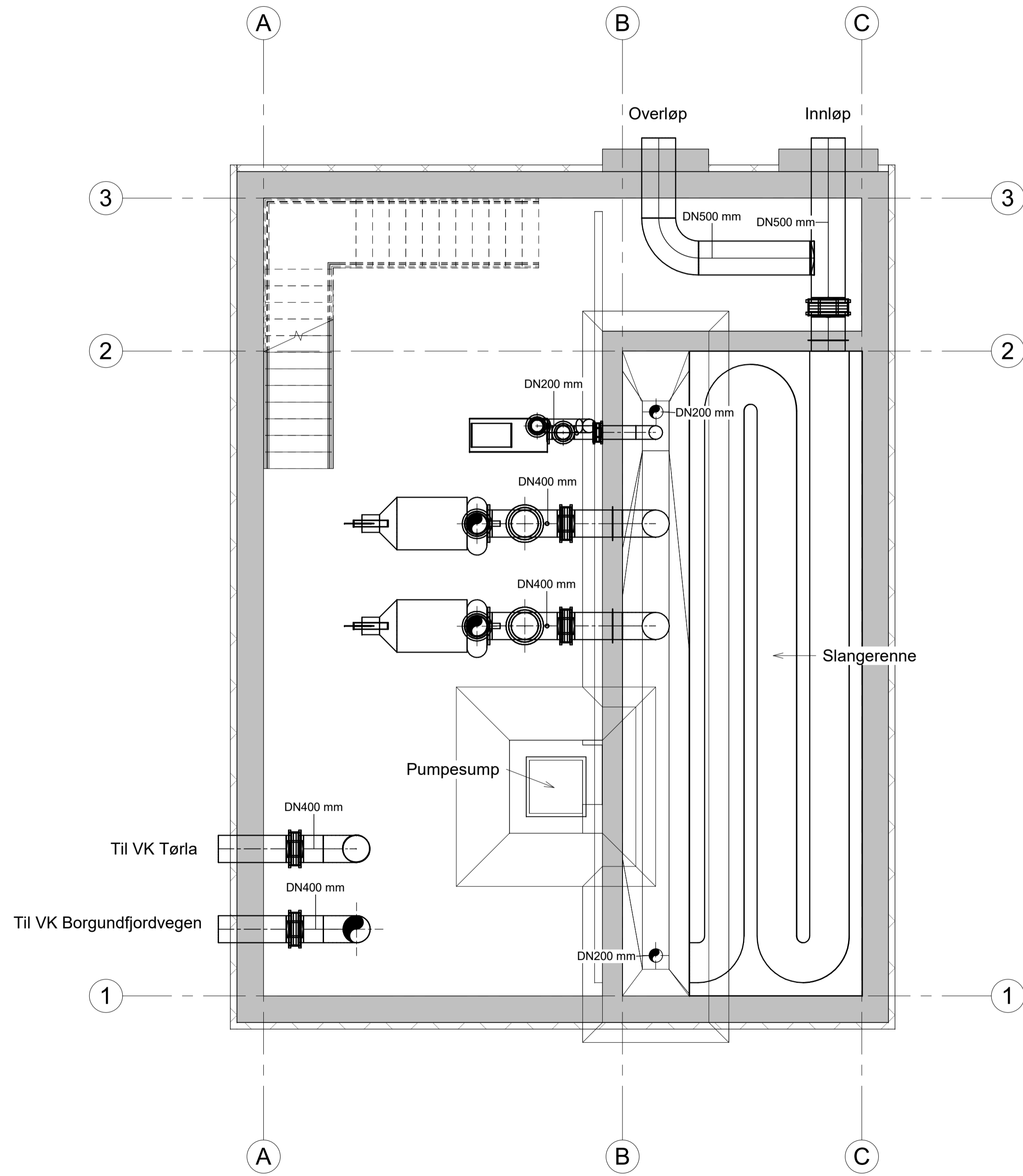
Plan U.ETG 1 : 50
