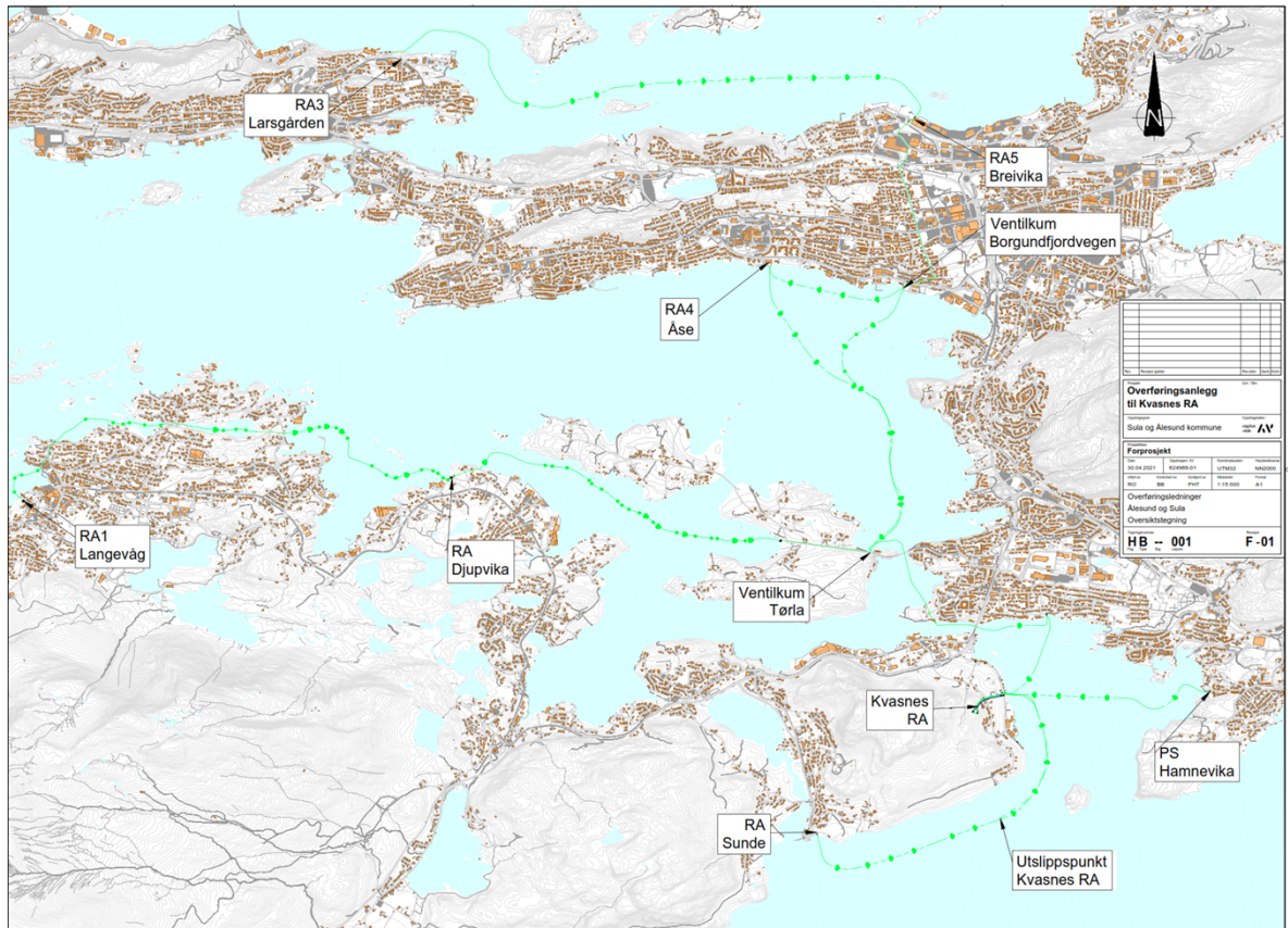
Figur 5-1: Oversiktskart for overføringsanlegg med sentrale installasjoner
