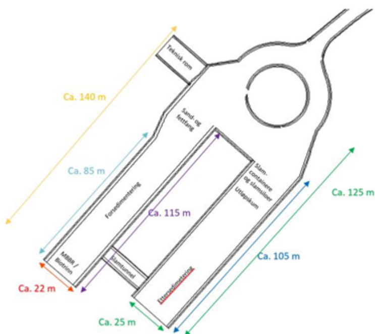
Figur 4-4 Dimensjoner fjellhaller
