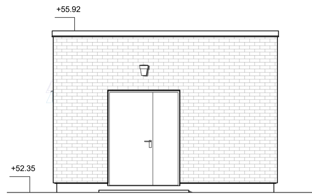
Sør 1 : 50
